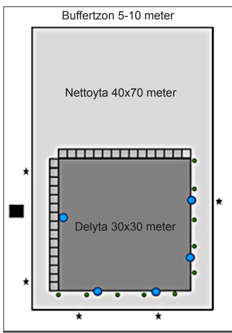
Figur 2. Obsytornas utformning.
