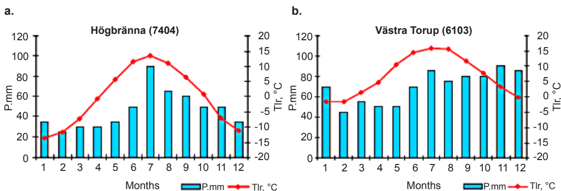
Figur 11. Exempel på meteorologiska data publicerade inom obsyteprogrammet. I diagrammen visas månadsnederbörd och månadsvisa luftmedeltemperaturer för Högbränna i Västerbotten (a) och Västra Torup i Skåne (b). Data är från närliggande SMHI-stationer och gäller perioden 1960-1990. Från Lundin och Lode (2007).
