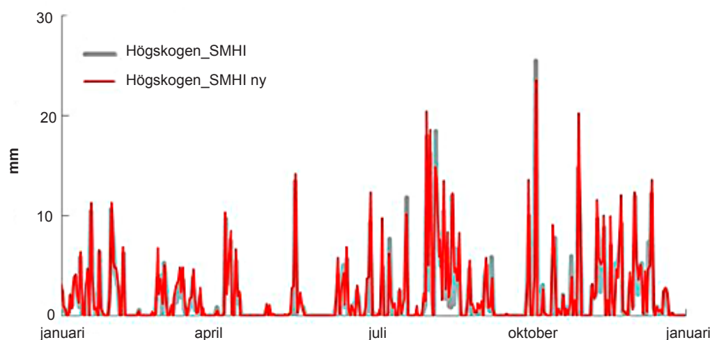
Figur 10. En jämförelse av dygnsmedelvärden för lufttemperatur (a) samt dygnsnederbörd (b) under året 2008 vid Högslogen, mellan de värden som beräknats från lokala mätningar (kallas "lokal"), de som laddats ner från SMHI's LuftWebb (kallas "SMHI ny") för de koordinater som gäller för ytan, samt de värden som tidigare beräknats från närliggande SMHI stationer (kallas "SMHI").
